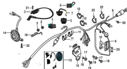
FIG. 20 SISTEMA ELECTRICO
