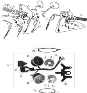
FIG. 10 MANGOS, SWITCH Y TABLERO
