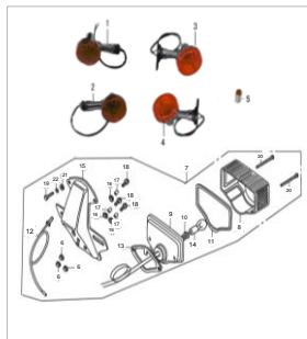
FIG.19 PIDEVIAS Y STOP
