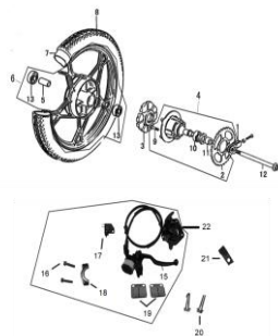
FIG.13 LLANTA TRASERA Y FRENO DELANTERO
