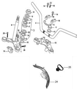
FIG. 11 T DE BARRAS, TIMON Y LODERA DELANTERA
