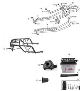
FIG. 16 PARRILLAS TRASERAS, FILTRO DE AIRE Y BATERIA
