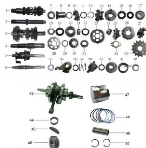
FIG. 7 TRANSMISION, CIGÜEÑAL Y PISTON
