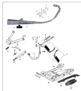
FIG. 17 ESCAPE, PATA DOBLE Y MULETA
