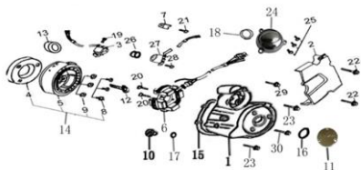
FIG. 7 MAGNETO
