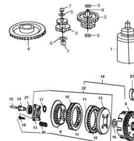
FIG. 6 MOTOR DE ESTARTER Y CLUTCH
