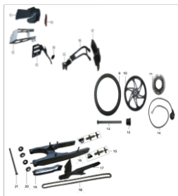
FIG. 16 LODERA TRASERA, LLANTA DELANTERA Y MULETA
