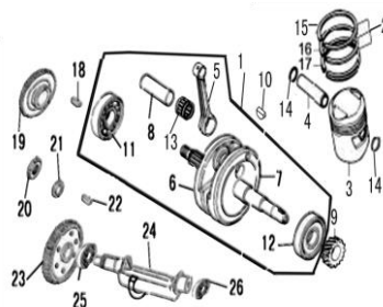
FIG. 8 CIGÜEÑAL Y PISTON
