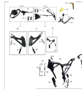
FIG. 18 SISTEMA DE FRENOS, POSAPIES Y CHASIS
