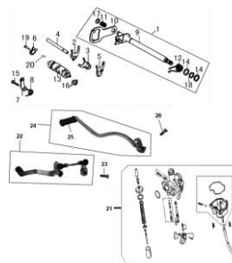
FIG. 11 SISTEMA DE CAMBIOS, CARBURADOR Y PALANCAS
