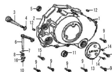
FIG. 3 TAPA DE CARTER RH
