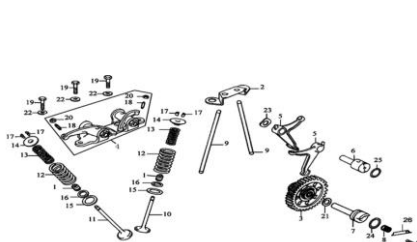
FIG. 2 EJE DE LEVAS Y VALVULAS
