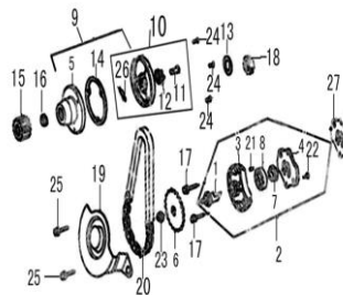
FIG. 5 BOMBA Y FILTRO DE ACEITE
