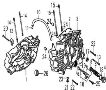
FIG. 4 CARTER
