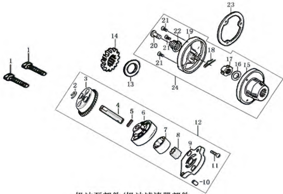
机油泵部件/机油滤清器部件 OIL PUMP/OIL FILTER
