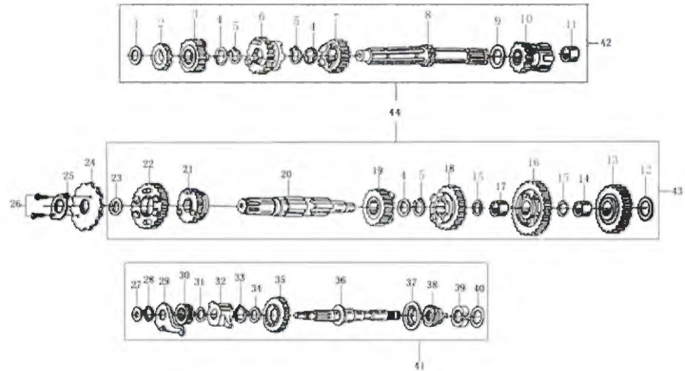
传动机构 TRANSMISSION MECHANISM
